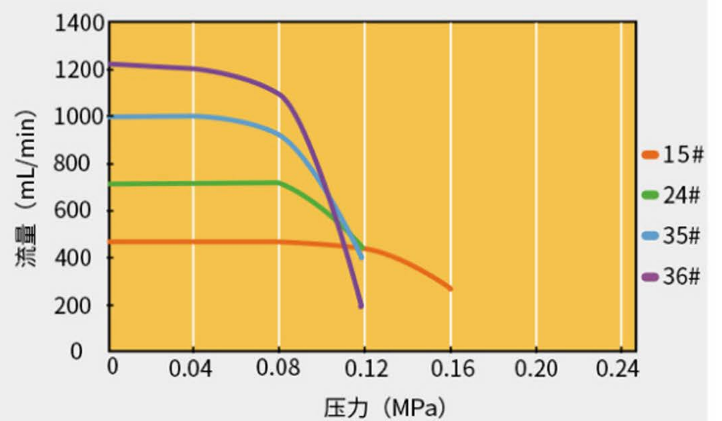
DY25泵头压力/流量曲线图 (100rpm)
